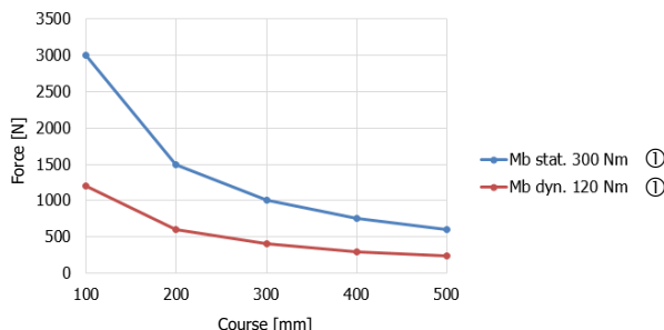
Moments de flexion de la Colonne de levage SE
