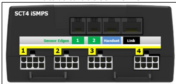
Boîte de contrôle SCT4 iSMPS
