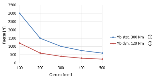
Momentos de flexión de la Columna de elevación SE
