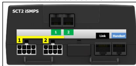
Boîte de contrôle SCT2 iSMPS
