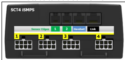
Boîte de contrôle SCT4 iSMPS
