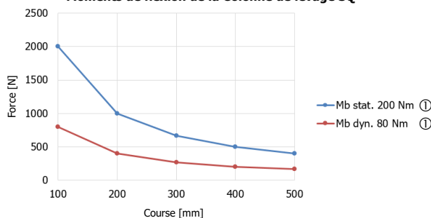
Moments de flexion de la Colonne de levage SQ
