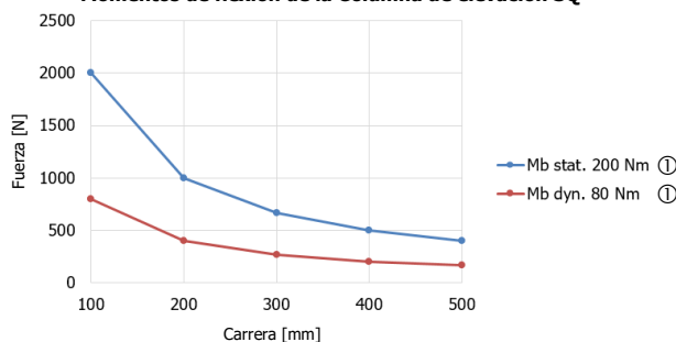
Momentos de flexión de la Columna de elevación SQ
