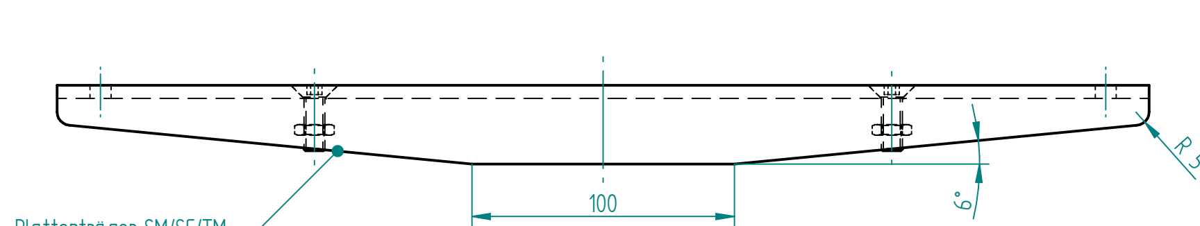
Plattenträger SM/SC/TM Table plate SM/SC/TM 127.00223 (4x)
